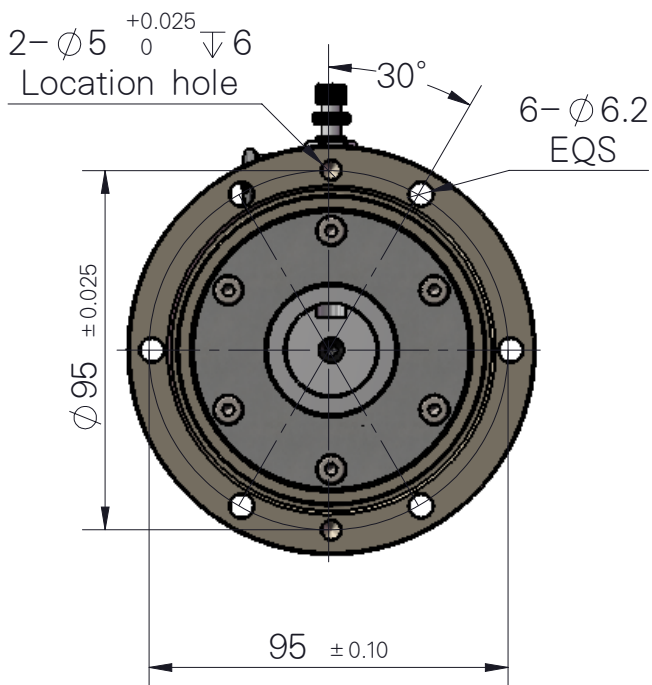
产品名称: 无限连续旋转接头-D95 型号: FY-CRJ-95-F
