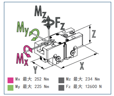
① 所示力矩和力为静态值, 适用于每个基爪, 且可能会同时出现。除抓取力自身产生的力矩外, 还可能产生负载。
